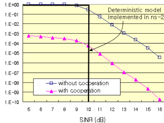
(b) FER versus SINR
